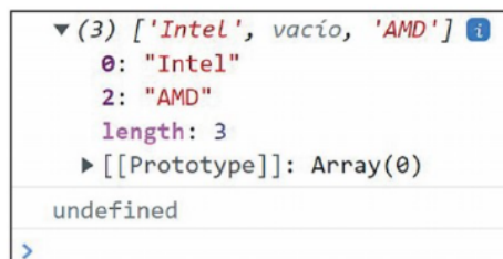
Figura 3.6. Aspecto de elementos undefined (vacío) en la consola de Google Chrome.
