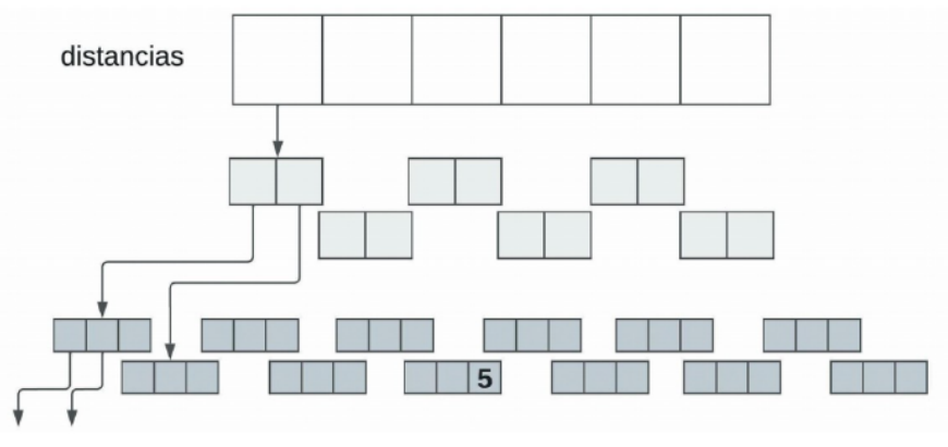
Figura 3.3. Diagrama conceptual de un array multidimensional.
